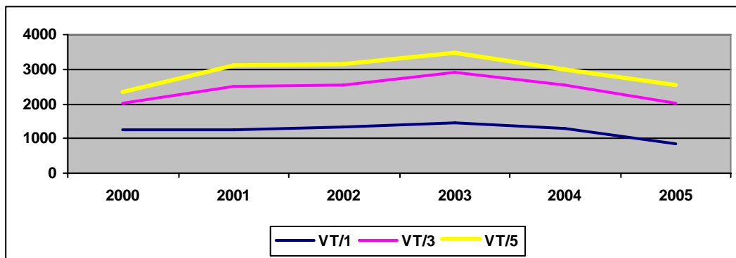
Fig. 14.5.2: Andamento delle iscrizioni all'Anagrafe Canina in tre delle cinque ASL
